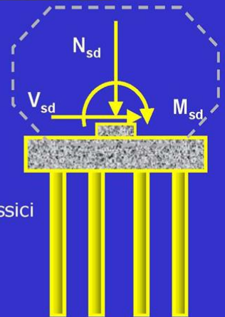
Azioni inerziali
